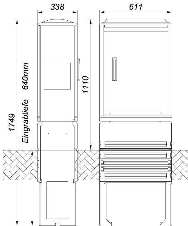
Abmessungen des A-Schranks Typ 2
