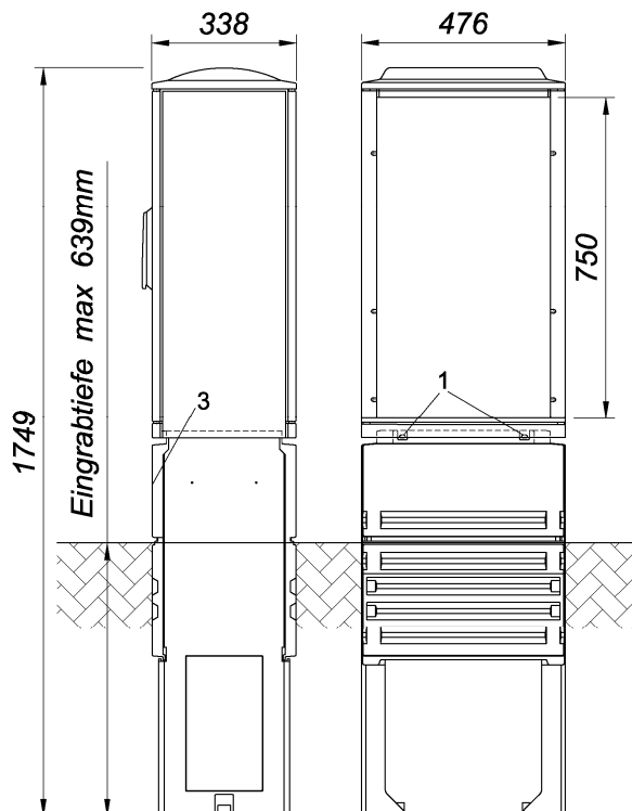
Abmessungen des A-Schranks Typ 1
